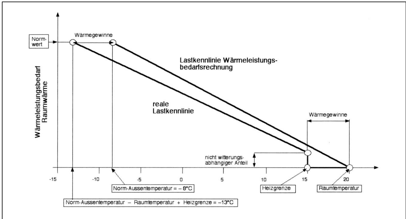
Abbildung 5: Berechnung der realen Lastkennlinie aus der Lastkennlinie gemäss Wärmeleistungsbedarfsrechnung durch Verschiebung um die Wärmegewinne nach links und einen nicht witterungsabhängigen Anteil nach oben.
