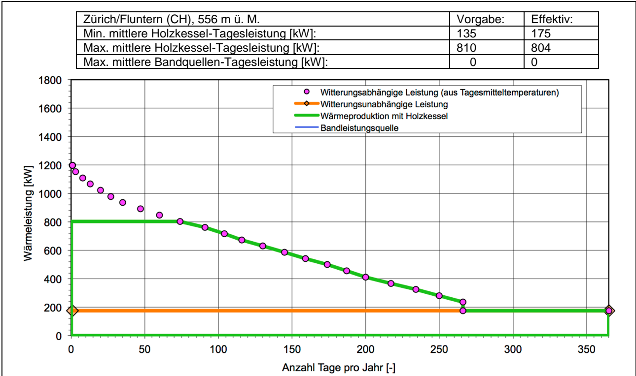
Abbildung 16: Jahresdauerlinie der benötigten Wärmeleistung mit umrahmten Holzessel-Anteil (grün) und Bandleistungs-Anteil (blau); Hinweis: die Wärmegewinne wurden schon in der Lastkennlinie berücksichtigt
