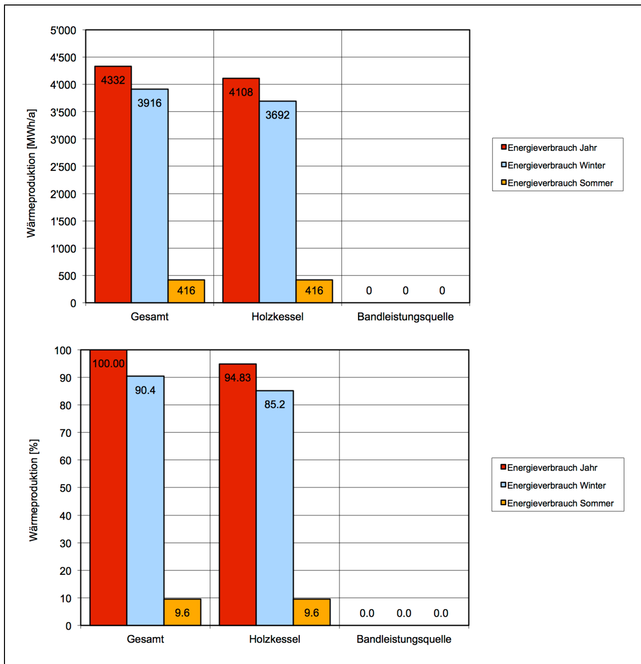
Abbildung 18: Gesamt-Wärmeproduktion und Produktionsanteile Holzessel und Bandleistungsquelle in [MWh] (oben) und in [%] (unten); die Differenz «Gesamtanlage – (Holzkessel + Bandlastquelle)» muss fossil erzeugt werden
