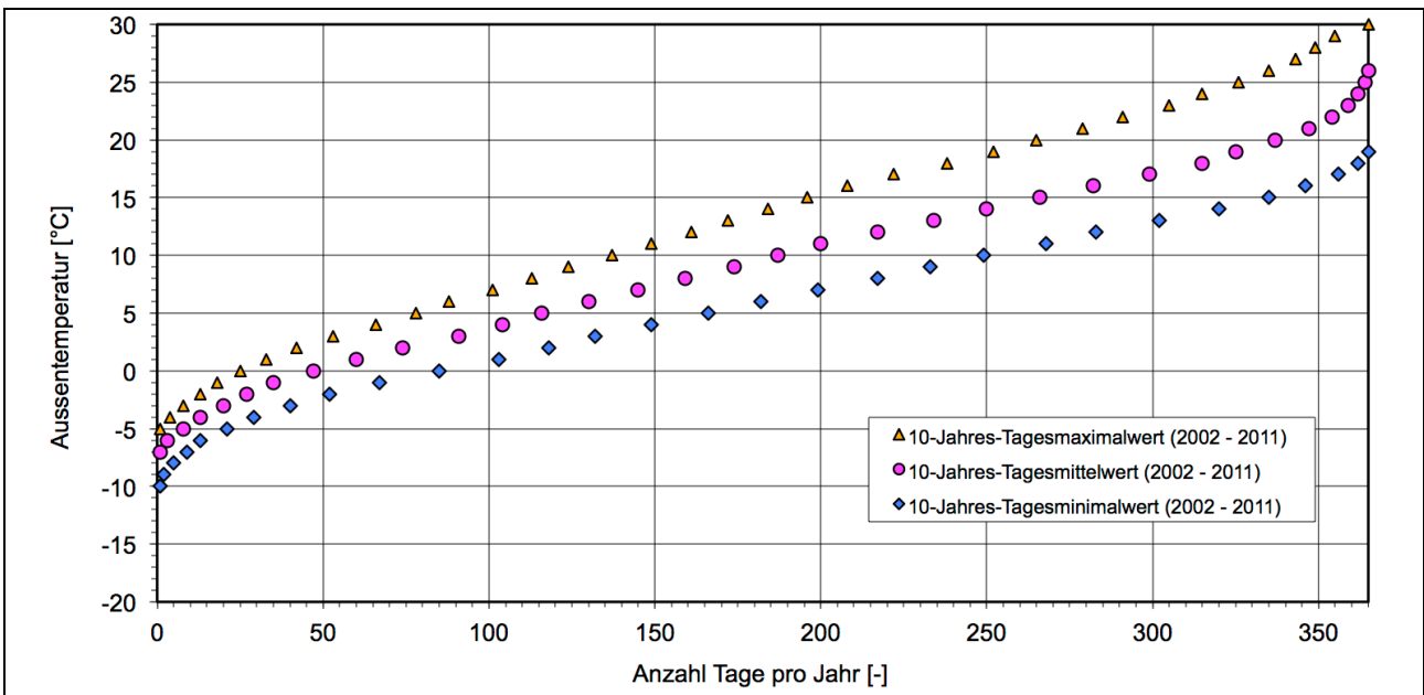
Abbildung 17: Jahresdauerlinien der Aussentemperatur (Zürich/Fluntern)
