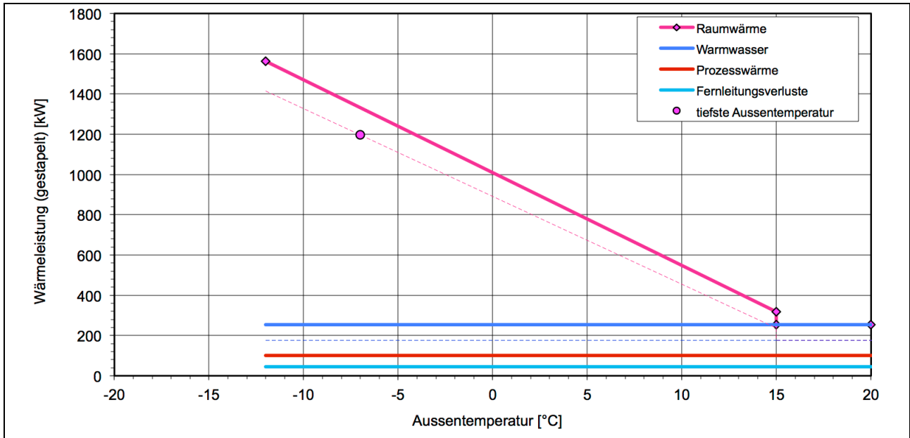
Abbildung 14: Ausgezogen die Lastkennlinie der Gesamtanlage; gestrichelt die gewichtete Lastkennlinie zur Berechnung der Jahresdauerlinie der benötigten Wärmeleistung
